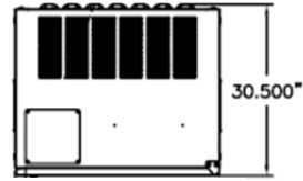
BRUA363078 Top View
